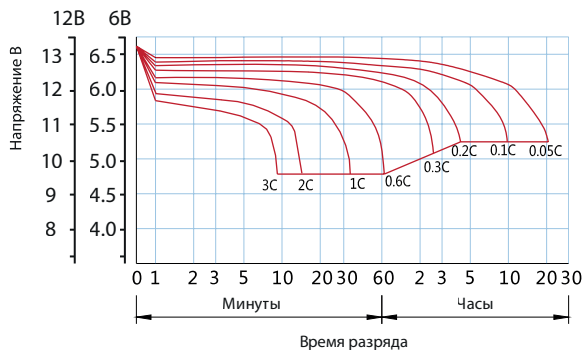
Характеристики заряда
